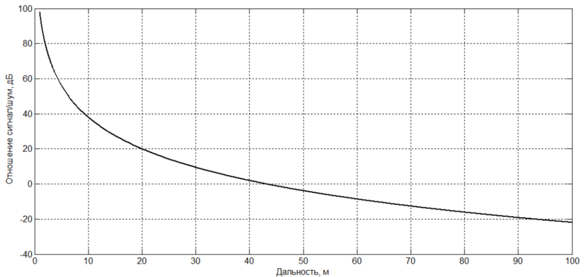
Рисунок 2.6 – Зависимость отношения «сигнал/шум» от дальности до НО при НО при n = 2 в свободном пространстве
