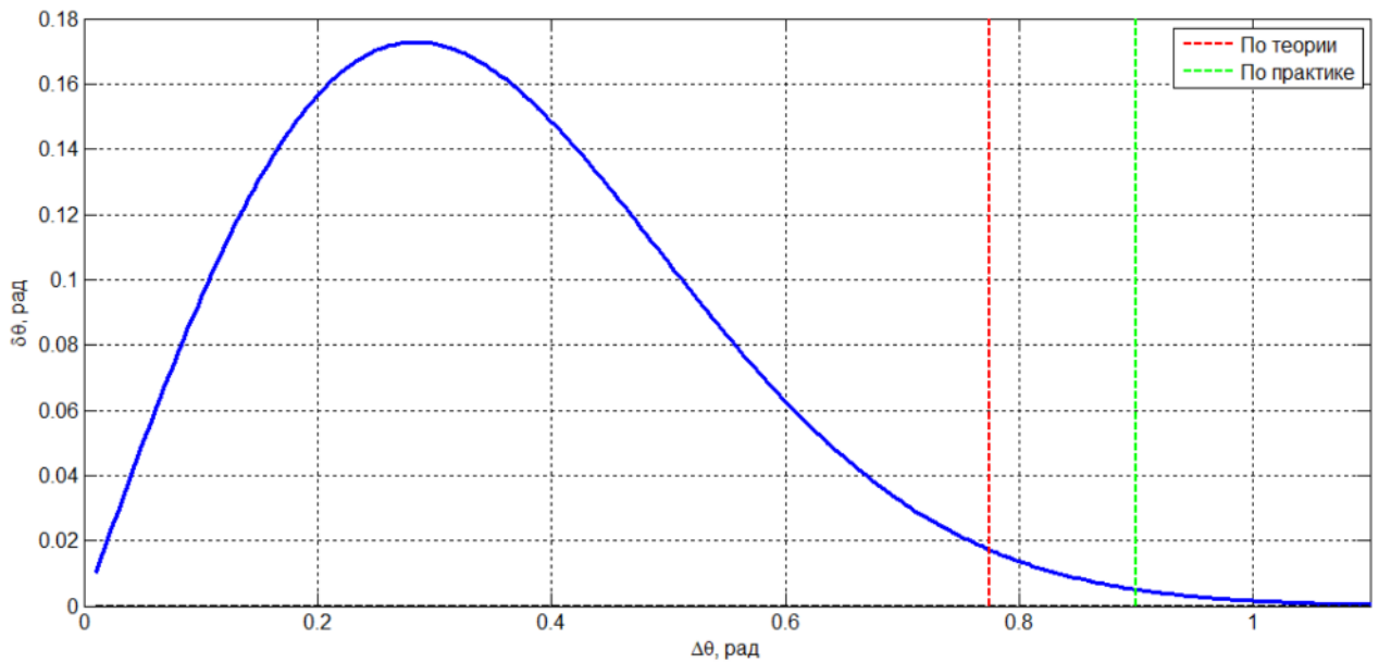
Рисунок 3.13 – Зависимость угловой погрешности от углового расстояния между двумя НО
