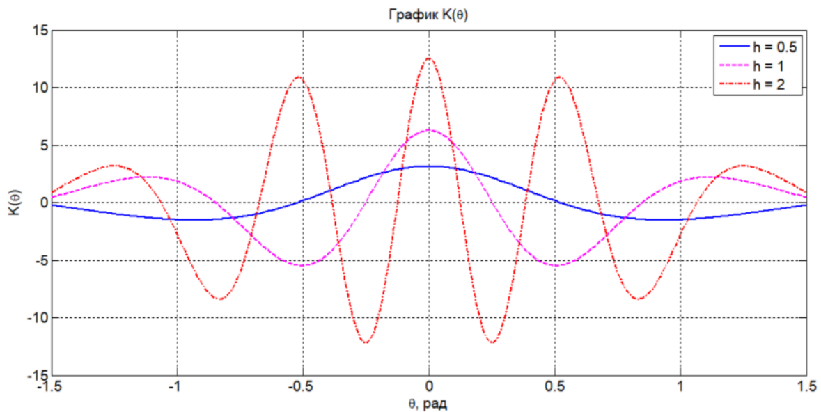
Рисунок 3.12 – Зависимость угловой локализации НО от параметра h при реализации фазового метода в нелинейной РТС
