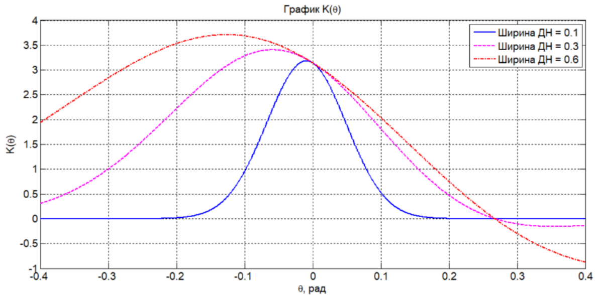
Рисунок 3.7 – Зависимость угловой локализации НО от ширины ДНА при реализации амплитудного метода (по методу минимума)
