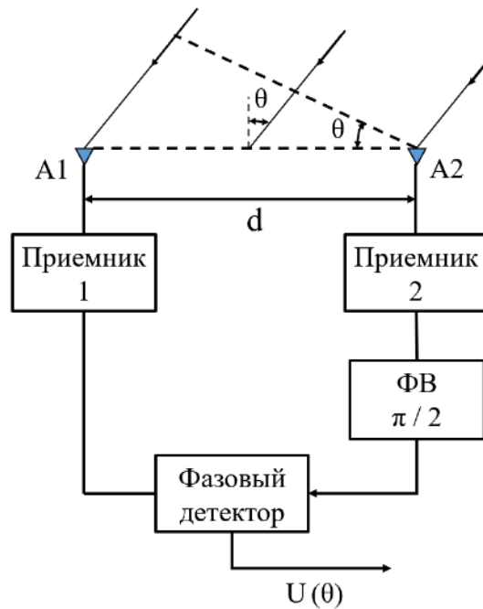
Рисунок 3.10 – Схема фазовой локализации угла прихода радиоволны от неоднородности с квадратичной ВАХ
