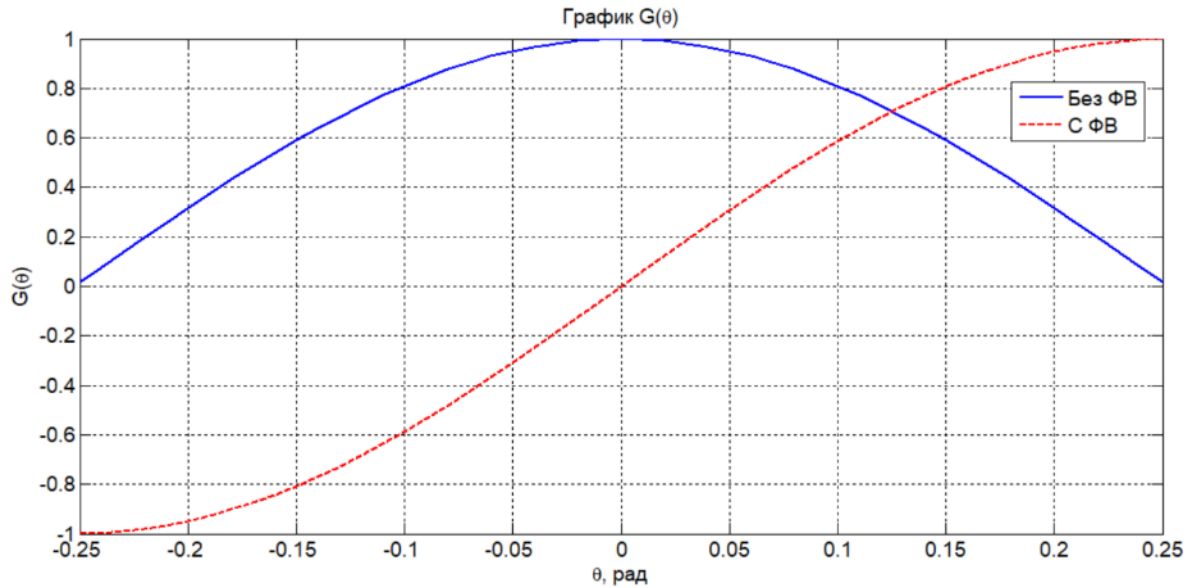
Рисунок 3.11 – Угловая характеристика фазового метода без фазовращателя и с фазовращателем
