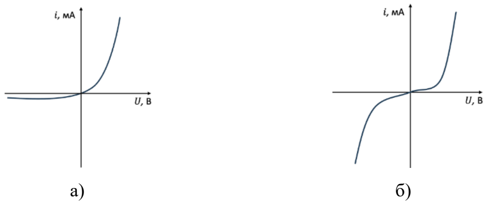
Рисунок 2.4 – ВАХ р-п перехода (а) и контакта металл-диэлектрик-металл (б)
