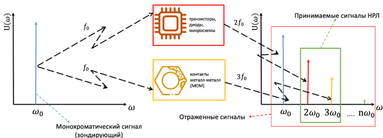
Рисунок 2.3 – Процесс нелинейного преобразования радиосигналов
