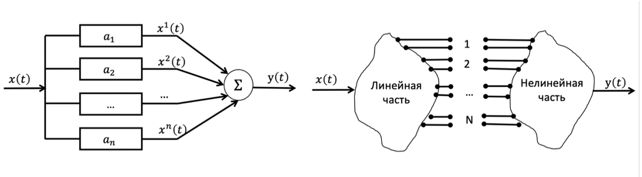
Рисунок 2.1 – Математическая и структурная модель описания точечного рассеивателя НО, описываемая с помощью рядов Тейлора
