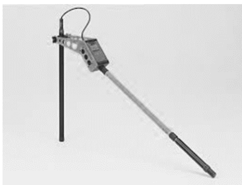
Магнитометр (регистратор магнитных аномалий, модель FOERSTER FEREX 4.032, Германия)
