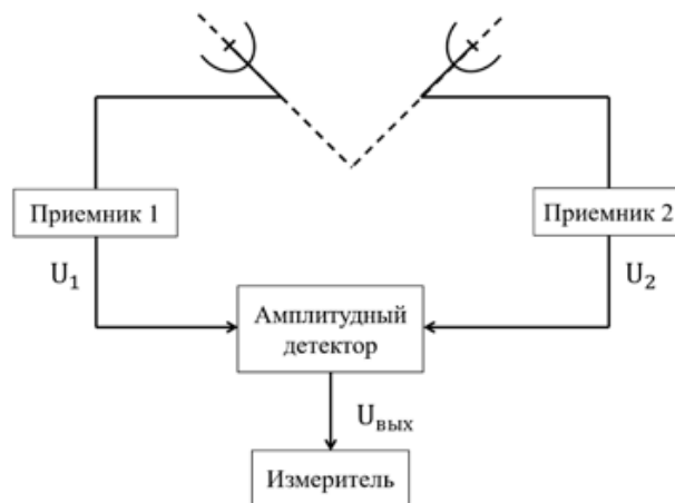
Рисунок 3.8 – Схема угловой локализации мобильной нелинейной РТС мониторинга с моноимпульсным методом сравнения
