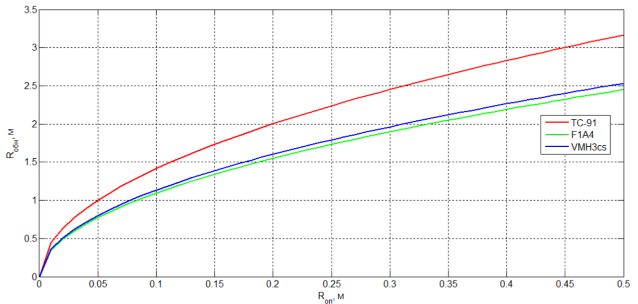
Рисунок 1.6 – Зависимости предельной глубины обнаружения объектов на сухом грунте ( \gamma_{сг} = 0.0001 См/м) от радиуса объекта поиска с различными приборами
