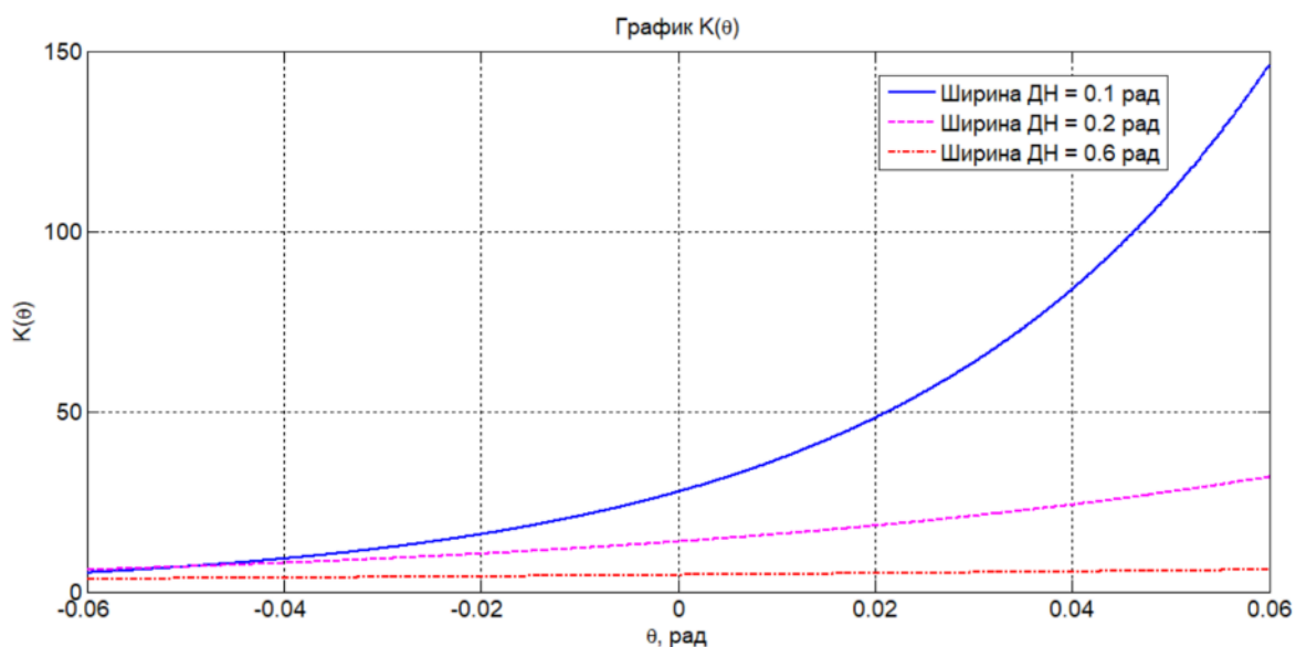
Рисунок 3.9 – Зависимость угловой локализации НО от ширины ДНА при реализации амплитудного метода (по методу сравнения)
